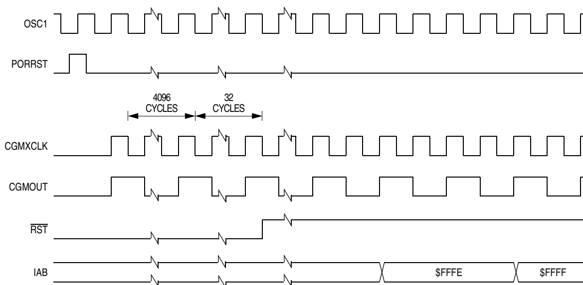
Figure 20-7. POR Recovery
