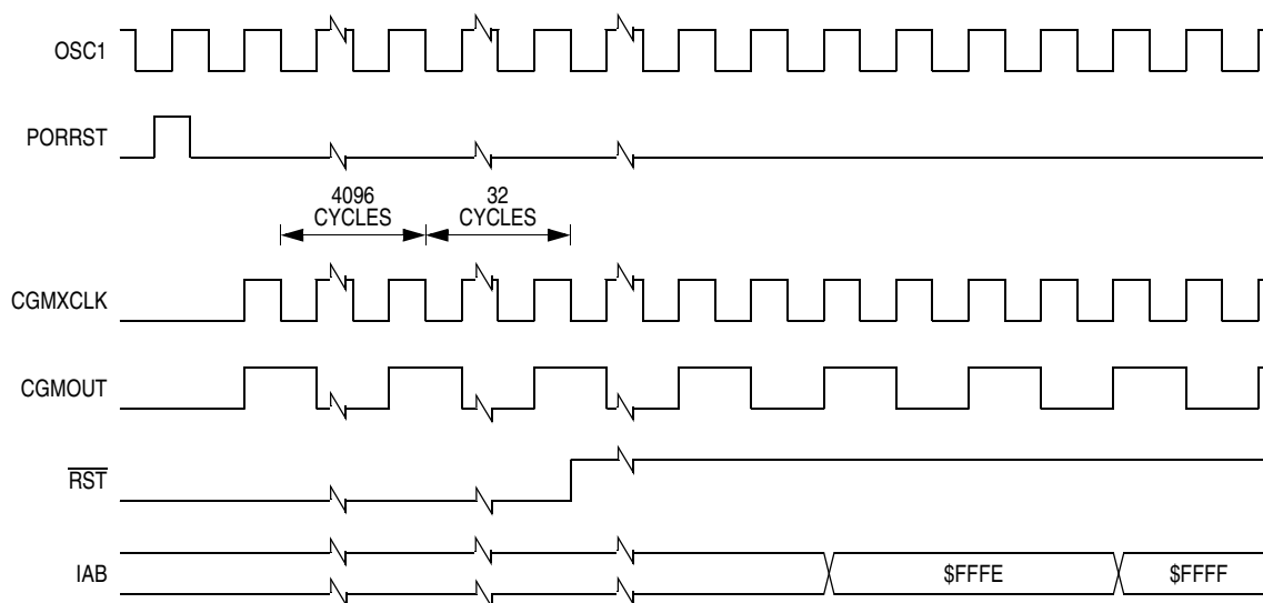
Figure 16-7. POR Recovery
