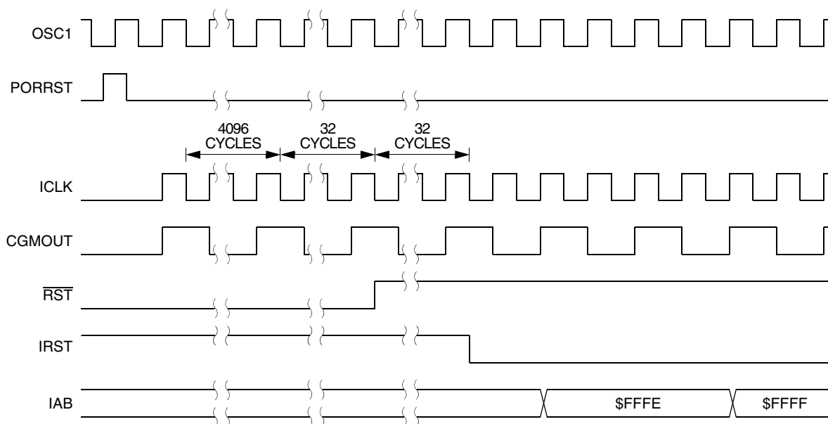
Figure 9-7. POR Recovery
