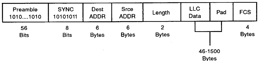
ISO 8802-3 (IEEE/ANSI 802.3) Data Frame
