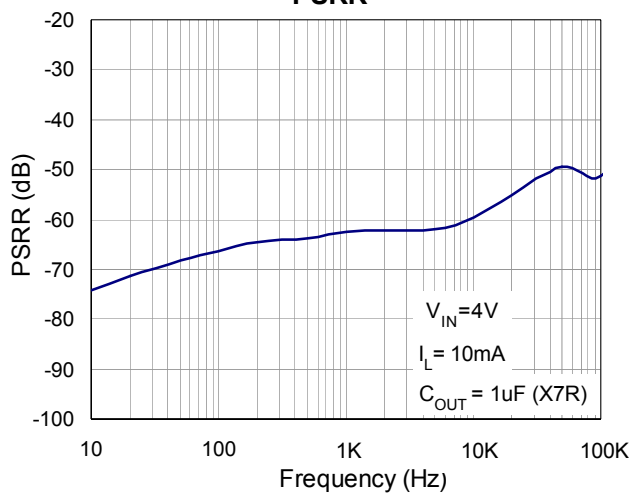
PSRR
