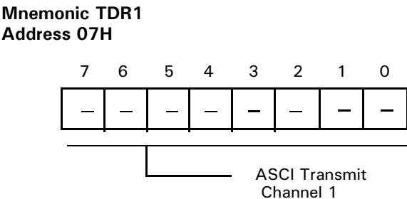
Figure 37. ASCI Register
