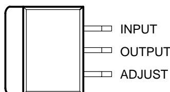
KTE PACKAGE (TOP VIEW)
