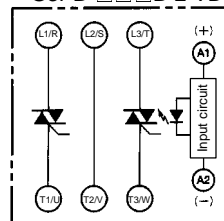
G3PB-□□□B-2-VD
