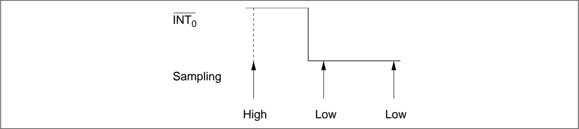
Figure 24 Edge Detection
