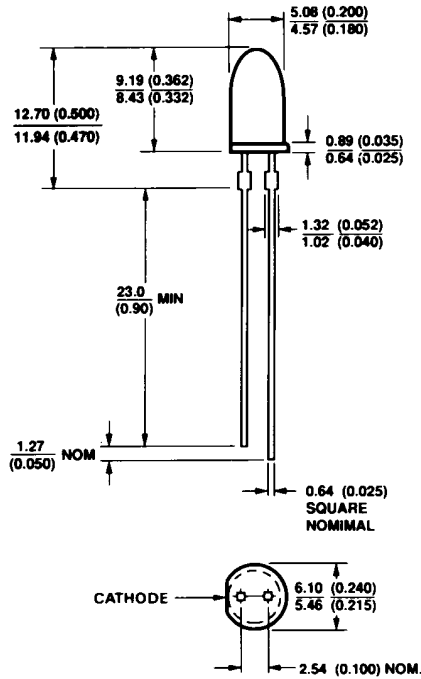
HLMP-8115/-8X05
