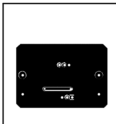
Fig. 25 Bottom Layer
