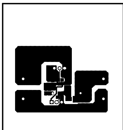
Fig. 24 Top Layer
