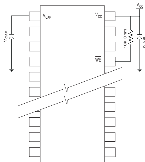
Figure 1. AutoStore Mode
