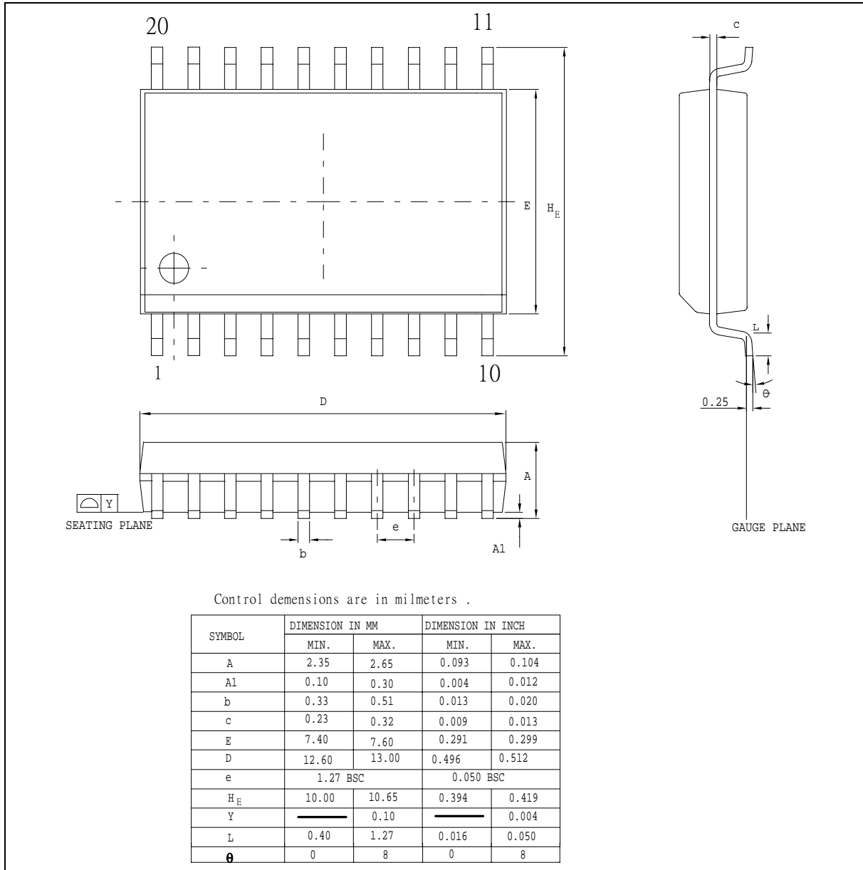
Figure 28-1: 20L SOP-300mil
