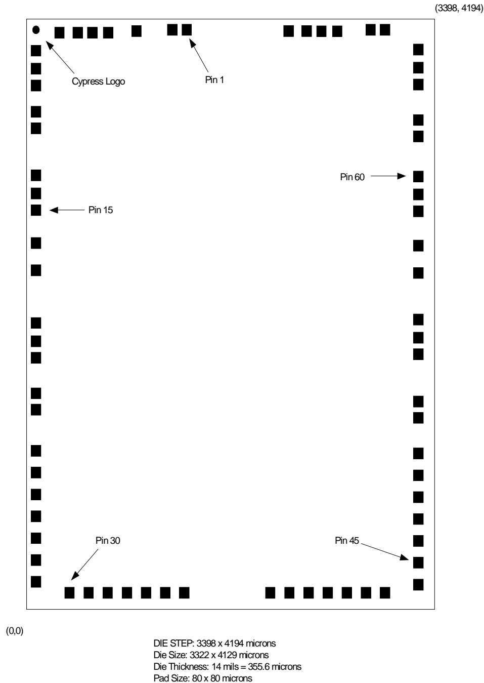
Figure 3-2. CY7C66113C DIE
