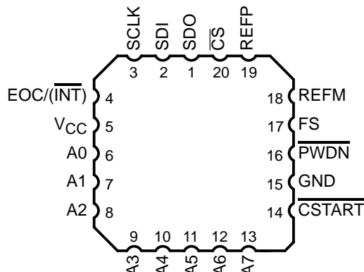
TLV2548M . . . FK PACKAGE
