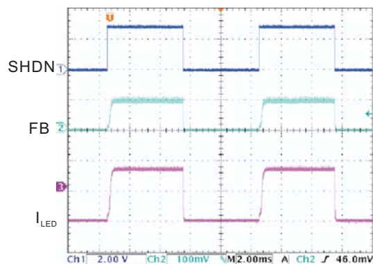
(3a) 100Hz
