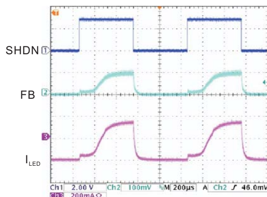
(3b) 1 KHz
