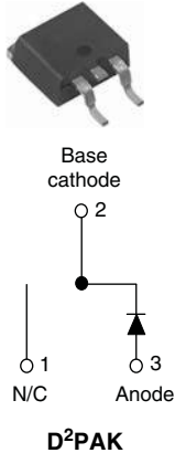
15ETH06SPbF
