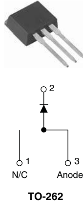
15ETH06-1PbF
